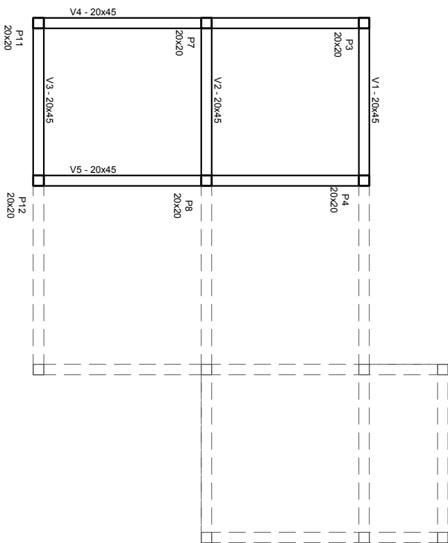
LOCAÇÃO EST. NÍVEL 1,99M - ESCADA NORTE
