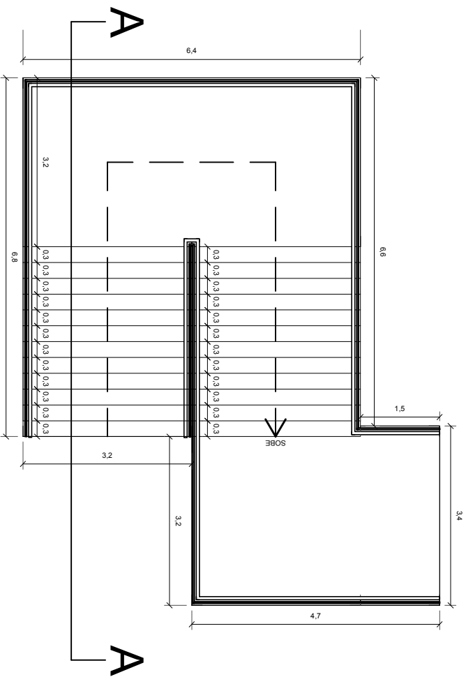
PLANTA BAIXA - ESCADA NORTE
